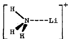
(51) C 3v
