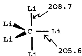
(15) D_{3h}
