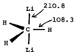
(27) D_{3h}
